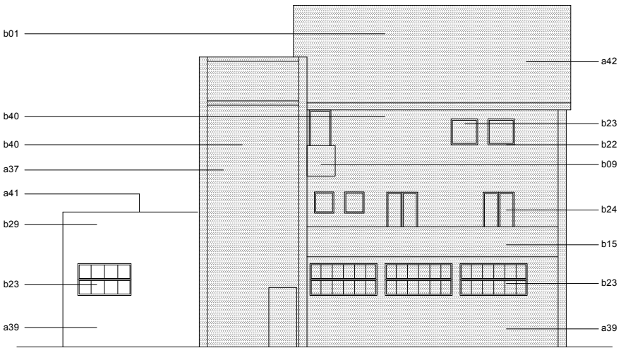
SEZIONE 3-3 (FRONTE SUD)
