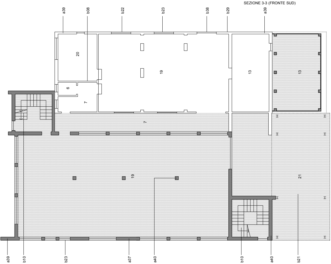
SEZIONE 3-3 (FRONTE SUD)
