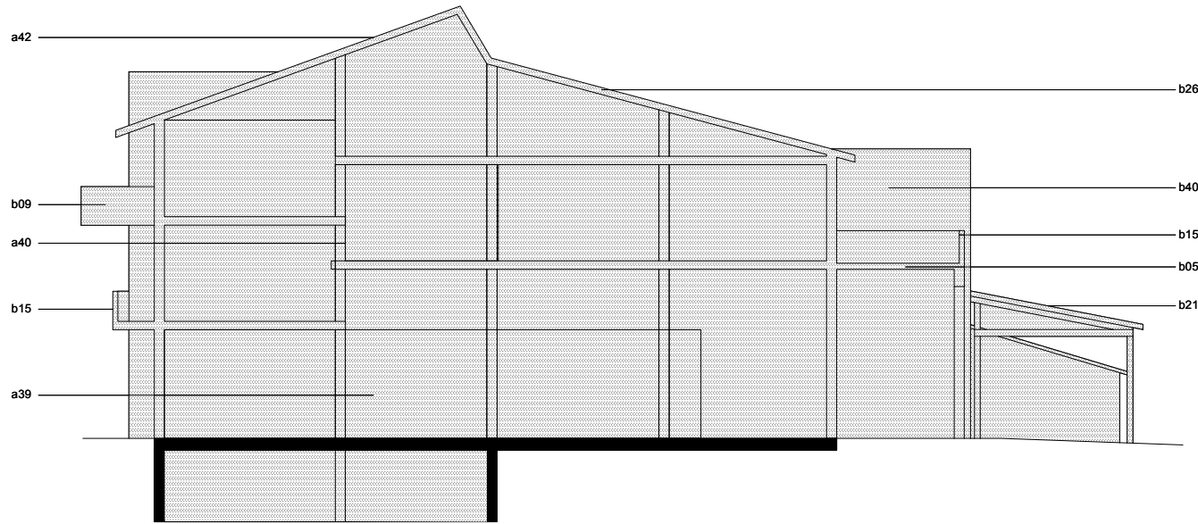
SEZIONE A-A
